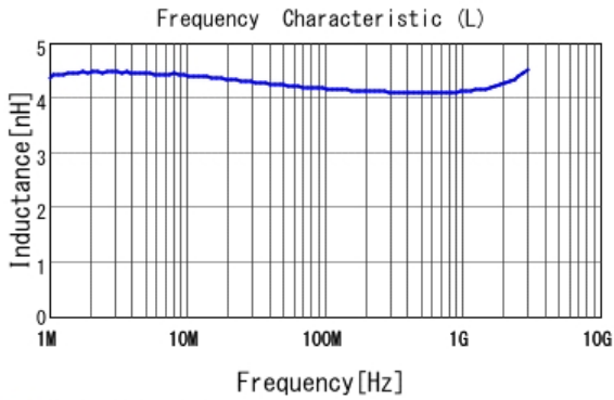
■ LQW15AN4N2G80 L
