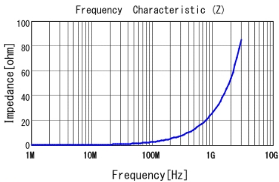
■ LQW15AN4N2G80 |Z|
