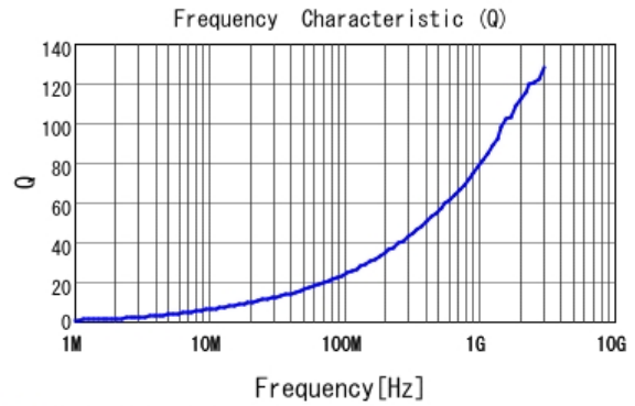
■ LQW15AN4N2G80 Q
