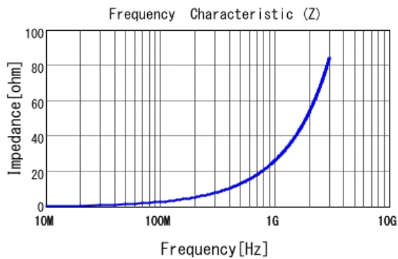
■ LQW15AN4N3B00 |Z|
