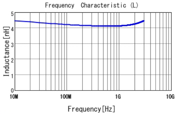
■ LQW15AN4N3B00 L
