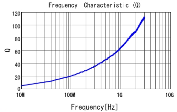
■ LQW15AN4N3B00 Q
