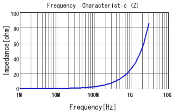
■ LQW15AN4N3B80 |Z|
