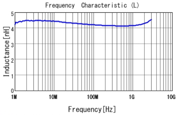
■ LQW15AN4N3B80 L
