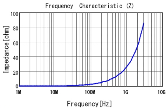
■ LQW15AN4N3G80 |Z|
