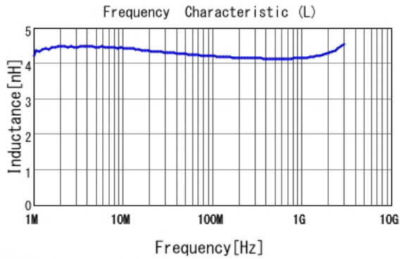
■ LQW15AN4N3G80 L
