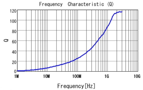
■ LQW15AN4N3G80 Q
