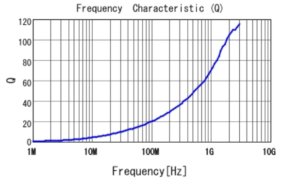
■ LQW15AN4N4G80 Q
