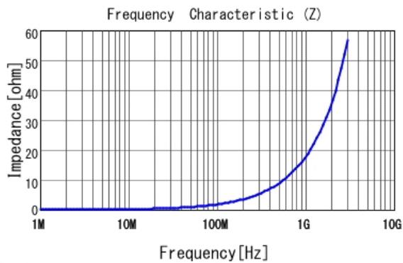
■ LQW15AN4N4G80 |Z|
