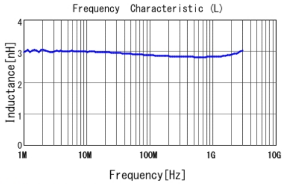
■ LQW15AN4N4G80 L
