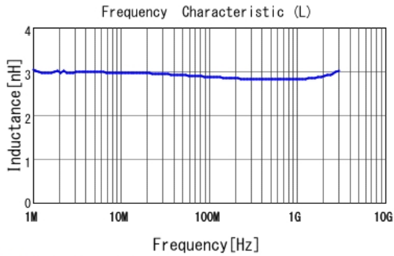
■ LQW15AN4N5G80 L
