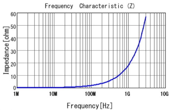
■ LQW15AN4N5G80 |Z|
