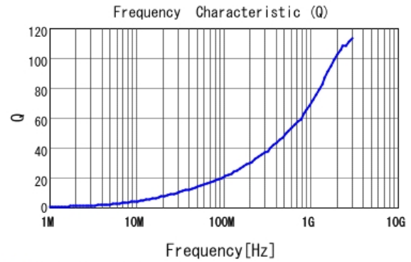
■ LQW15AN4N5G80 Q
