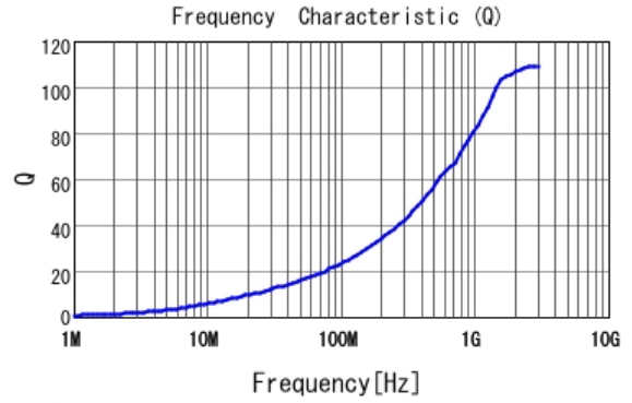
■ LQW15AN4N6G80 Q
