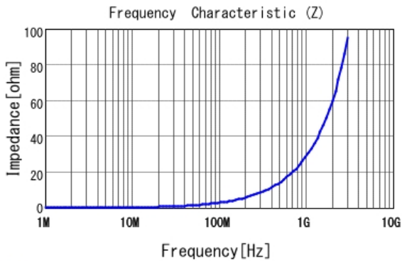
■ LQW15AN4N6G80 |Z|
