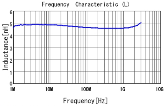
■ LQW15AN4N6G80 L
