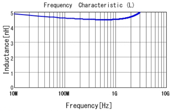
■ LQW15AN4N7B00 L
