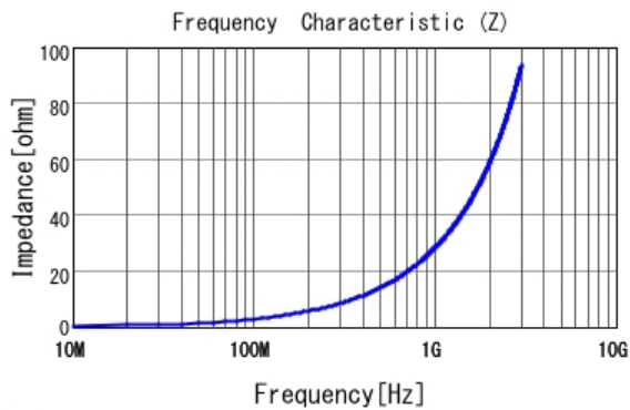
■ LQW15AN4N7B00 |Z|
