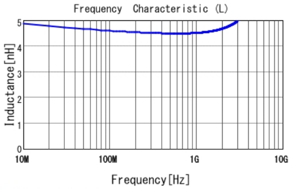
■ LQW15AN4N7C00 L
