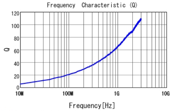
■ LQW15AN4N7C00 Q
