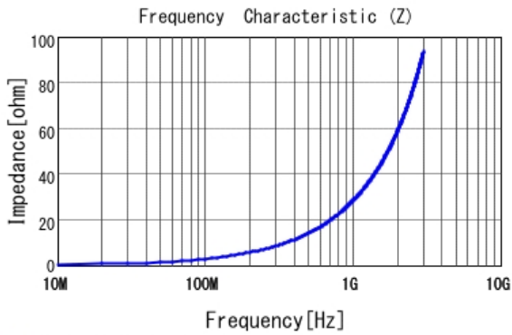
■ LQW15AN4N7C00 |Z|
