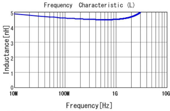
■ LQW15AN4N7D00 L
