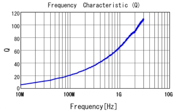
■ LQW15AN4N7D00 Q
