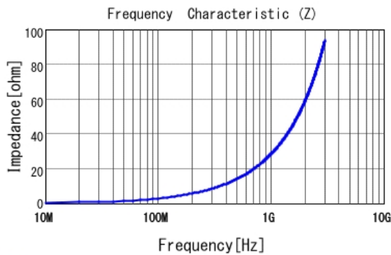
■ LQW15AN4N7D00 |Z|
