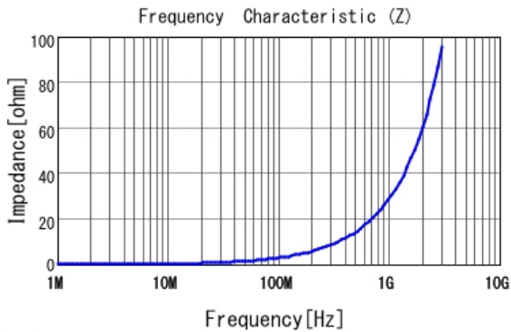
■ LQW15AN4N7G80 |Z|
