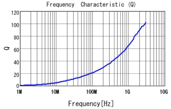
■ LQW15AN4N7G80 Q
