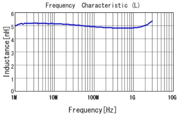
■ LQW15AN4N8G80 L
