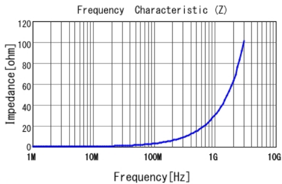
■ LQW15AN4N8G80 |Z|
