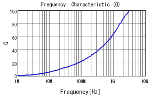
■ LQW15AN4N8G80 Q
