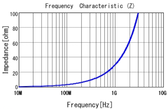
■ LQW15AN4N9B00 |Z|
