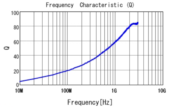
■ LQW15AN4N9B00 Q
