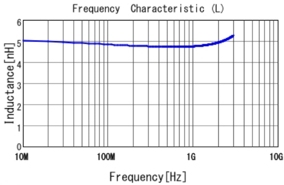
■ LQW15AN4N9B00 L
