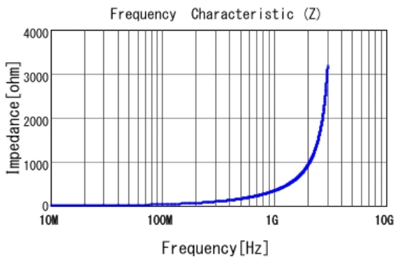
■ LQW15AN51NG00 |Z|
