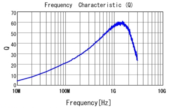
■ LQW15AN51NG00 Q
