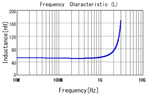
■ LQW15AN51NJ00 L
