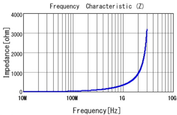
■ LQW15AN51NJ00 |Z|
