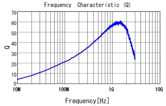
■ LQW15AN51NJ00 Q
