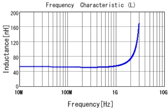
■ LQW15AN51NJ0Z L
