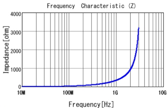
■ LQW15AN51NJ0Z |Z|
