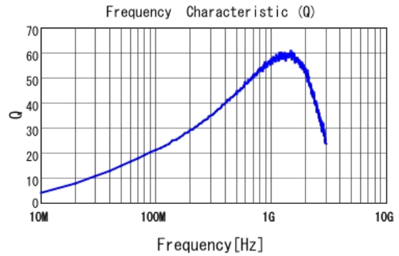
■ LQW15AN51NJ0Z Q
