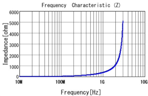
■ LQW15AN56NG00 |Z|
