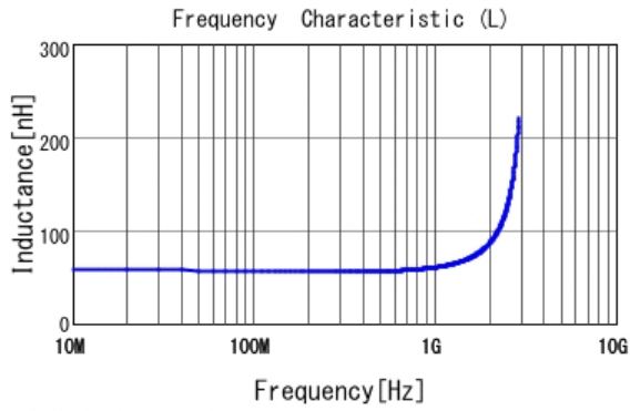
■ LQW15AN56NG00 L
