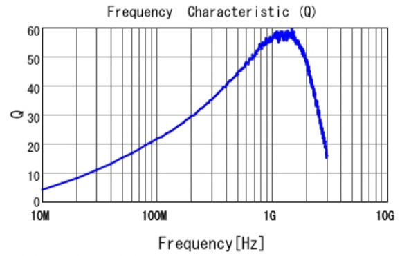
■ LQW15AN56NG00 Q
