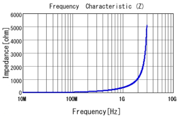
■ LQW15AN56NH00 |Z|
