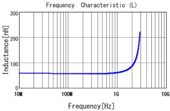
■ LQW15AN56NH00 L
