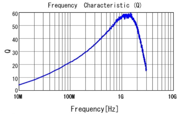
■ LQW15AN56NH00 Q
