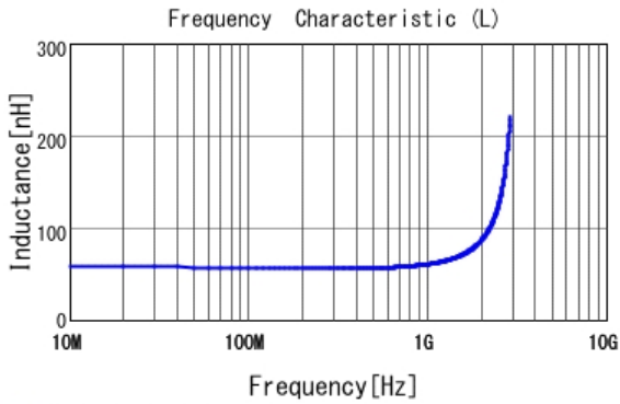
■ LQW15AN56NJ00 L
