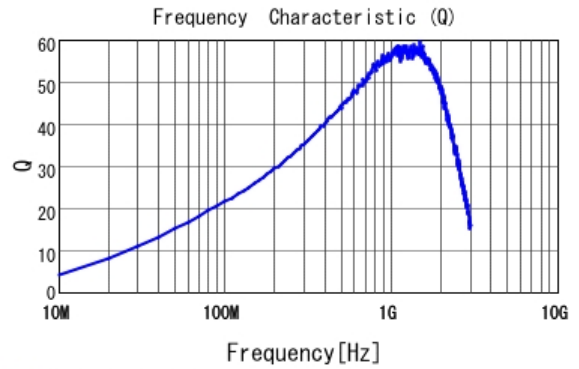
■ LQW15AN56NJ00 Q
