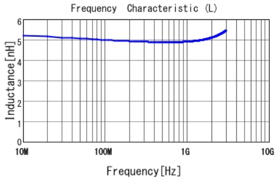
■ LQW15AN5N1B00 L
