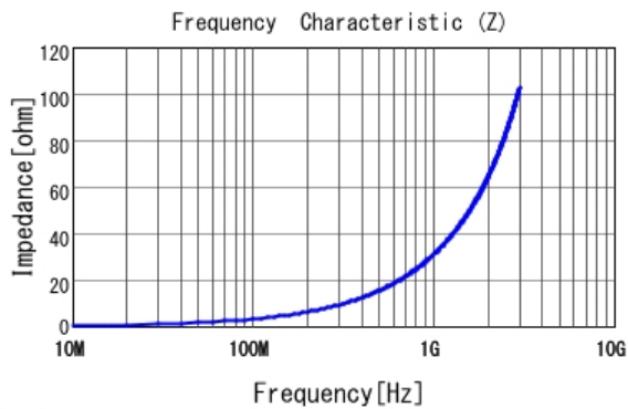
■ LQW15AN5N1B00 |Z|
