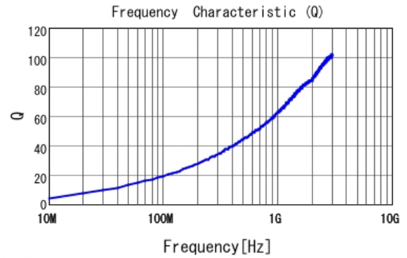
■ LQW15AN5N1B00 Q
