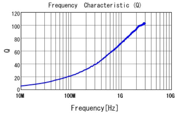
■ LQW15AN5N3C10 Q
