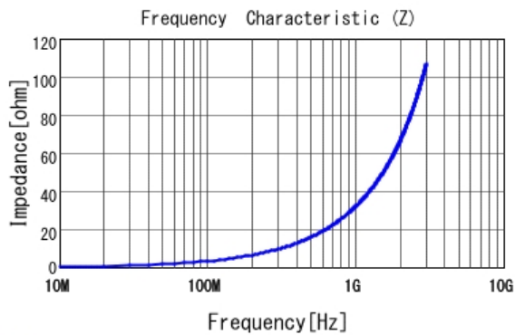
■ LQW15AN5N3C10 |Z|
