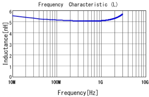
■ LQW15AN5N3C10 L
