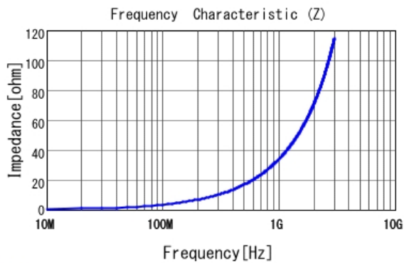
■ LQW15AN5N4C10 |Z|
