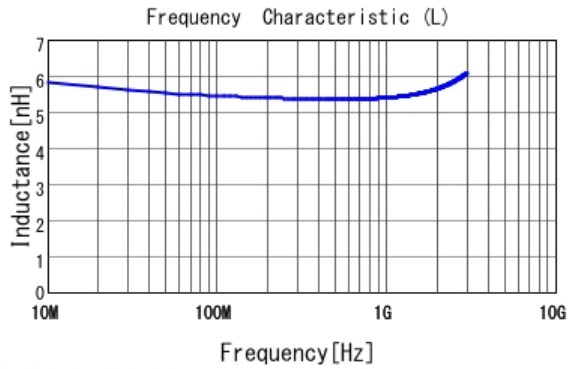
■ LQW15AN5N4C10 L
