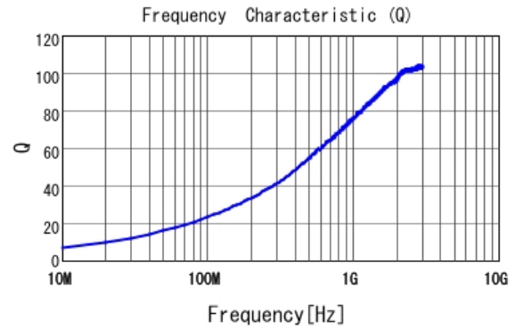
■ LQW15AN5N4C10 Q
