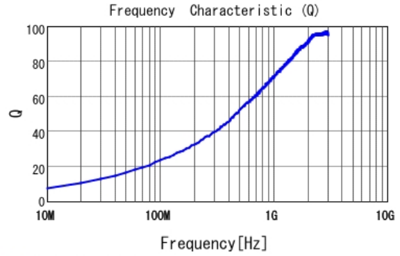
■ LQW15AN5N5C10 Q
