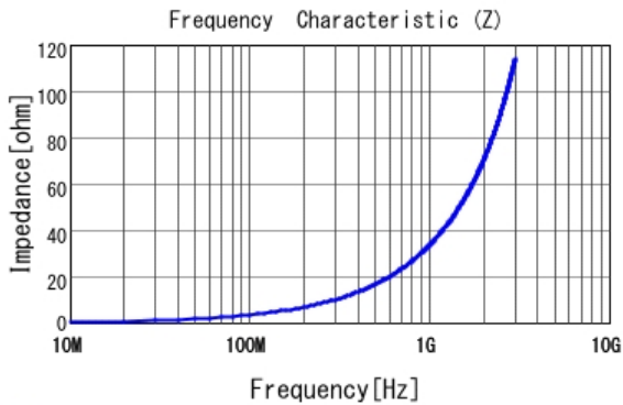
■ LQW15AN5N5C10 |Z|
