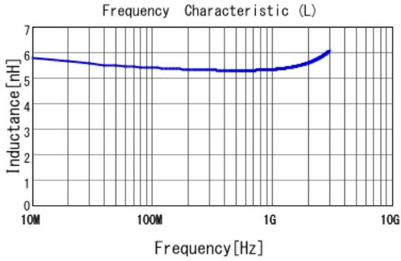
■ LQW15AN5N5C10 L
