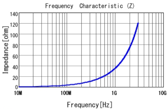
■ LQW15AN5N7C10 |Z|
