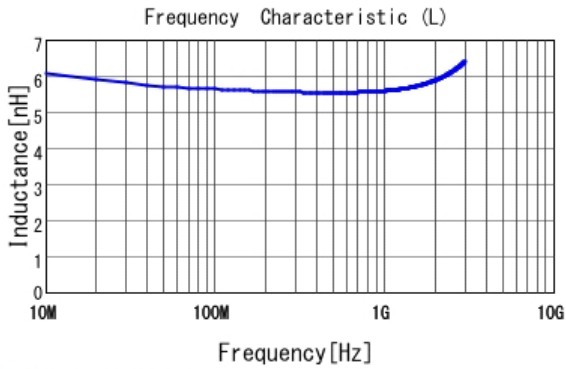
■ LQW15AN5N7C10 L
