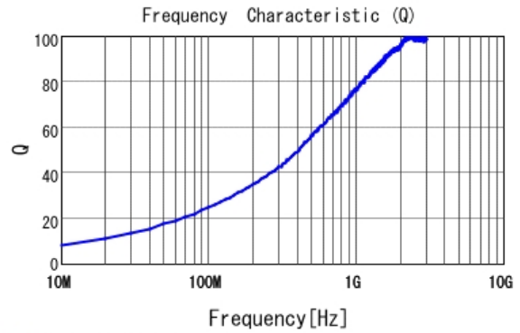
■ LQW15AN5N7C10 Q
