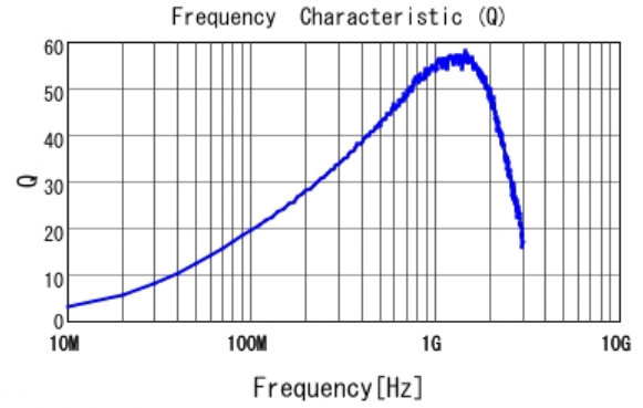
■ LQW15AN62NG00 Q
