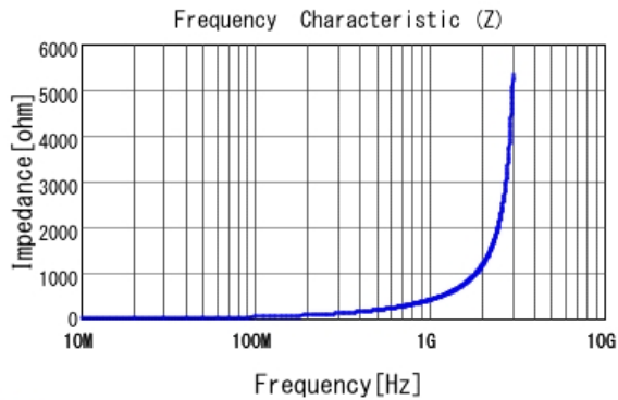
■ LQW15AN62NG00 |Z|
