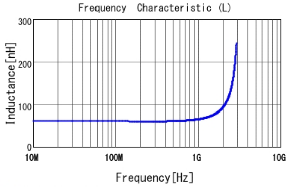
■ LQW15AN62NG00 L
