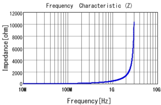
■ LQW15AN68NG00 |Z|
