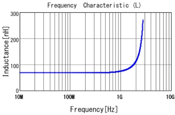
■ LQW15AN68NG00 L
