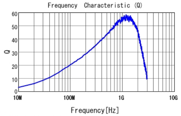
■ LQW15AN68NG00 Q
