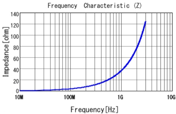
■ LQW15AN6N0C10 |Z|
