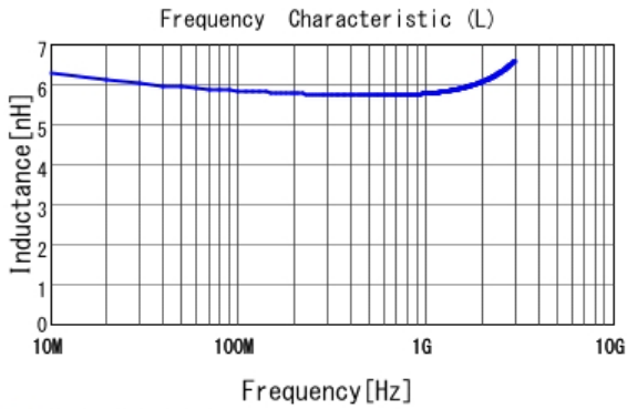
■ LQW15AN6N0C10 L
