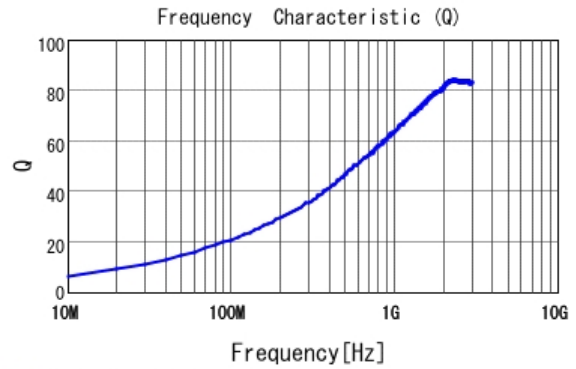
■ LQW15AN6N1C10 Q
