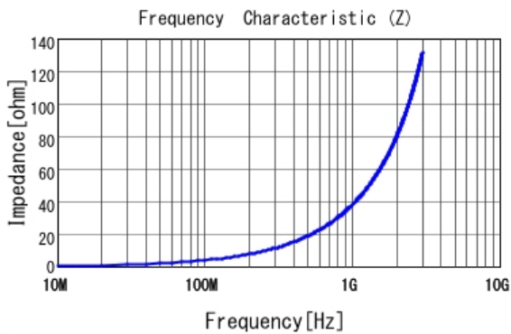
■ LQW15AN6N1C10 |Z|
