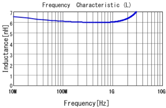
■ LQW15AN6N1C10 L
