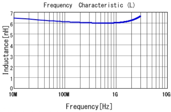
■ LQW15AN6N2B00 L
