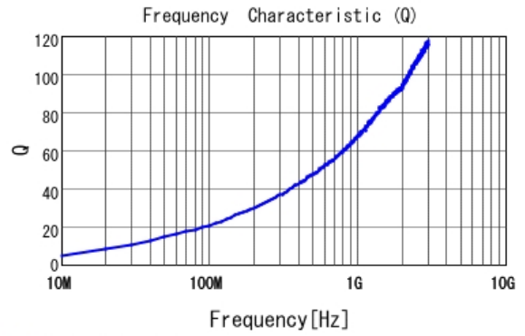
■ LQW15AN6N2B00 Q
