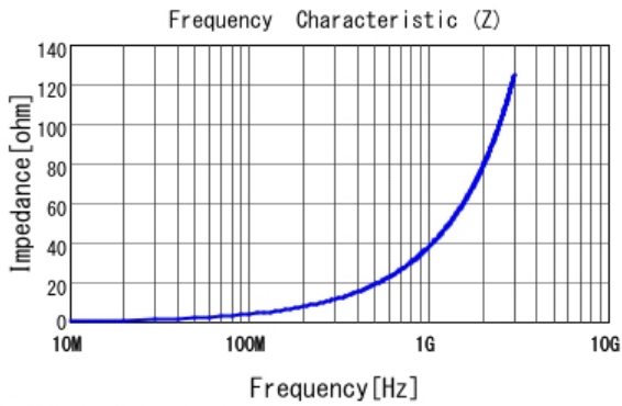
■ LQW15AN6N2B00 |Z|
