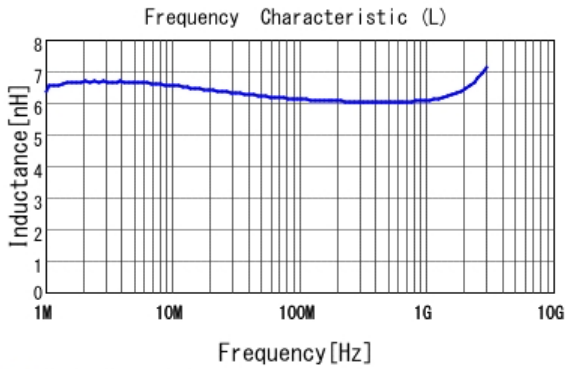
■ LQW15AN6N1B80 L
