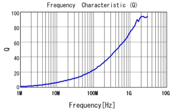
■ LQW15AN6N1B80 Q
