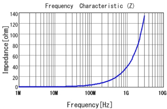
■ LQW15AN6N1B80 |Z|
