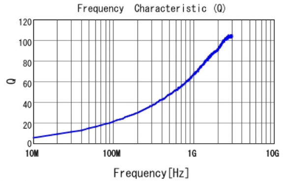
■ LQW15AN6N8G00 Q
