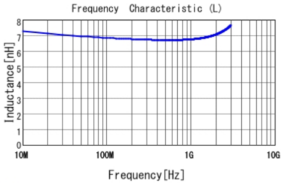
■ LQW15AN6N8G00 L
