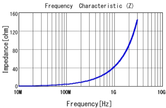
■ LQW15AN6N8G00 |Z|
