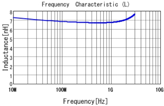
■ LQW15AN6N8H00 L
