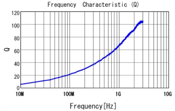
■ LQW15AN6N8H00 Q
