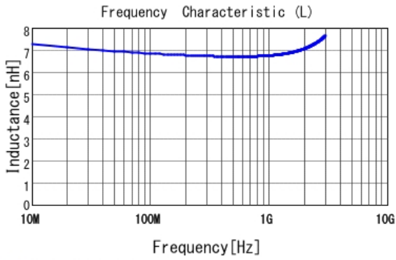
■ LQW15AN6N8J00 L
