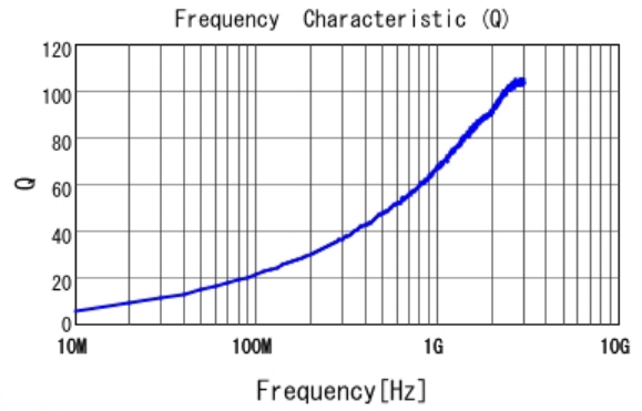
■ LQW15AN6N8J00 Q
