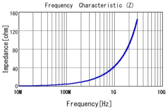
■ LQW15AN6N8J00 |Z|
