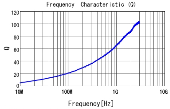
■ LQW15AN7N3G00 Q
