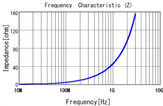
■ LQW15AN7N3G00 |Z|
