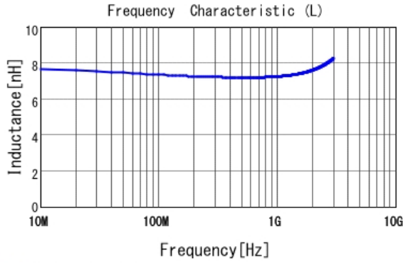
■ LQW15AN7N3G00 L
