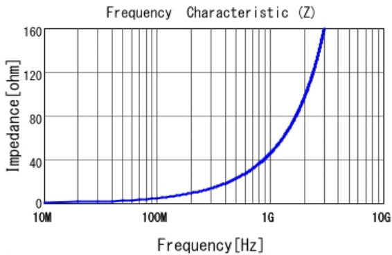
■ LQW15AN7N4C10 |Z|
