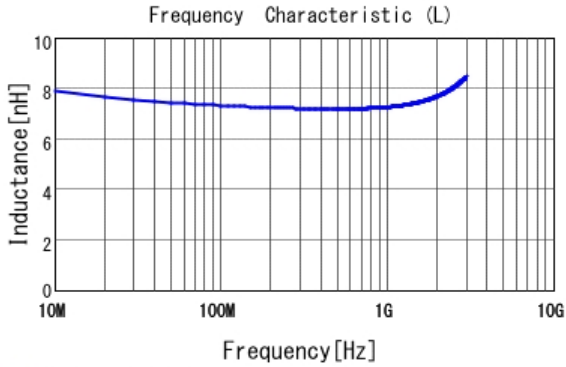
■ LQW15AN7N4C10 L
