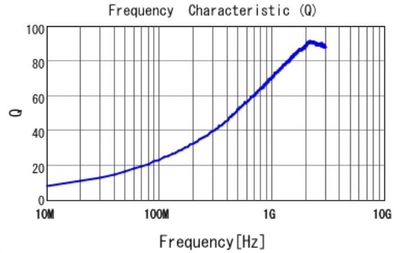
■ LQW15AN7N4C10 Q
