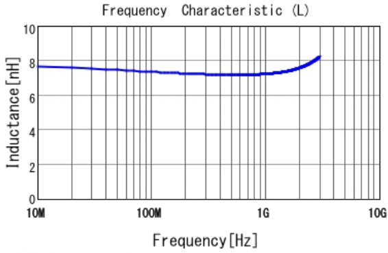
■ LQW15AN7N5G00 L
