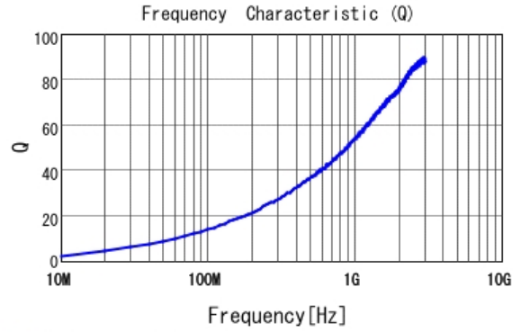
■ LQW15AN7N5G00 Q
