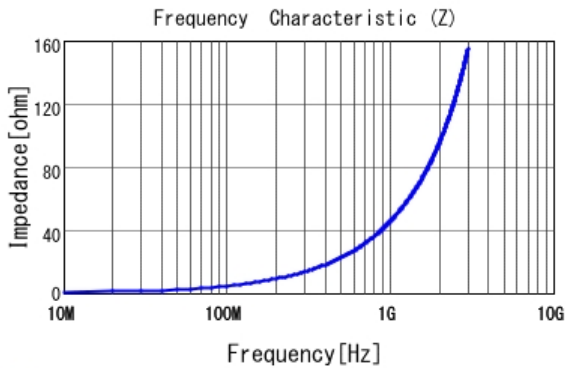
■ LQW15AN7N5G00 |Z|
