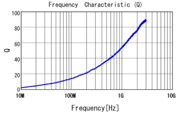
■ LQW15AN7N5H00 Q
