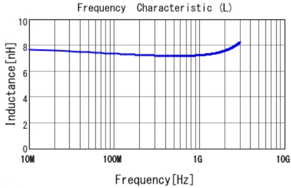
■ LQW15AN7N5H00 L
