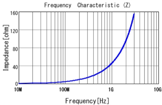
■ LQW15AN7N5H00 |Z|
