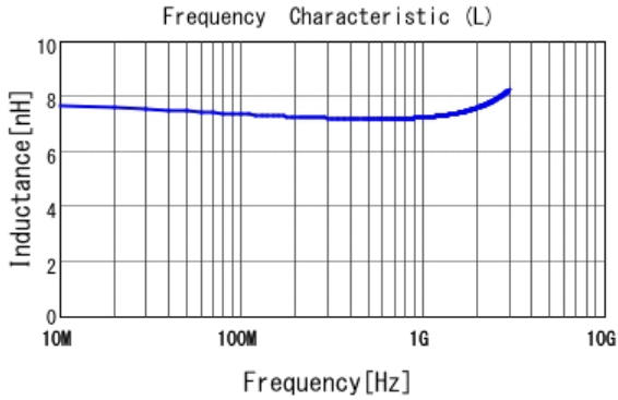
■ LQW15AN7N5J00 L
