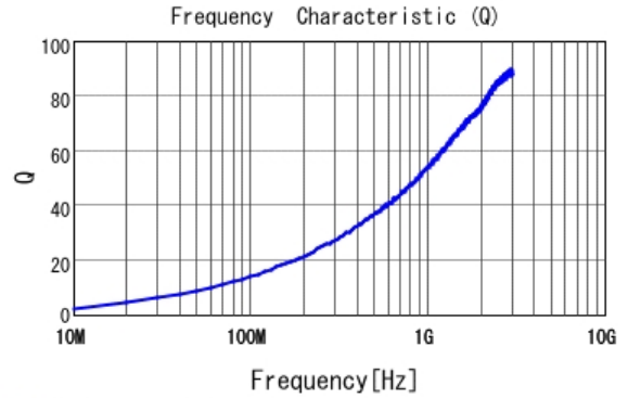
■ LQW15AN7N5J00 Q
