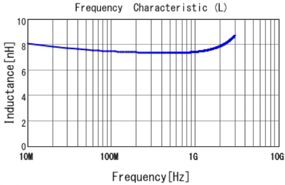
■ LQW15AN7N6C10 L
