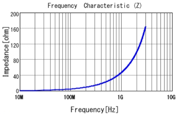
■ LQW15AN7N6C10 |Z|
