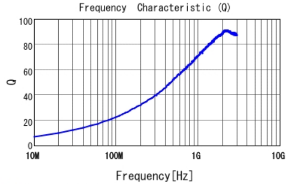
■ LQW15AN7N6C10 Q
