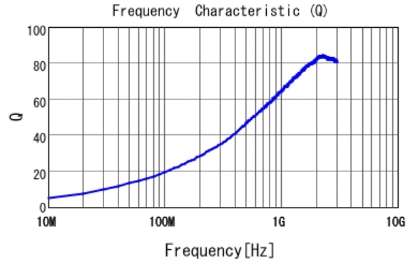
■ LQW15AN7N7C10 Q
