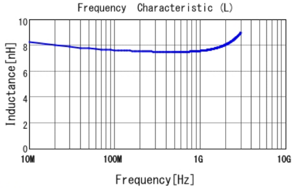
■ LQW15AN7N7C10 L
