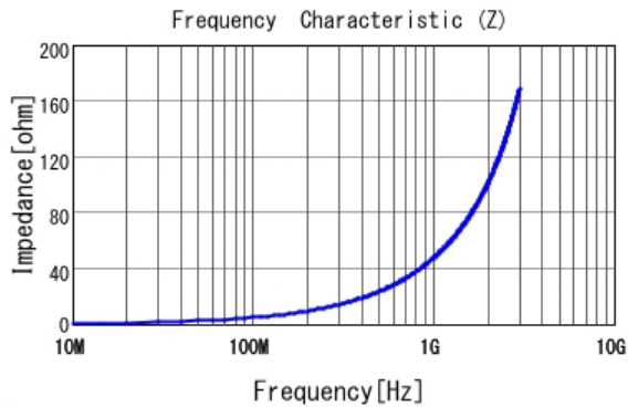
■ LQW15AN7N7C10 |Z|
