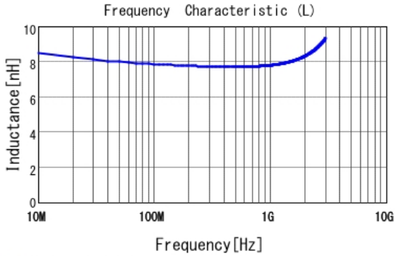
■ LQW15AN7N8C10 L
