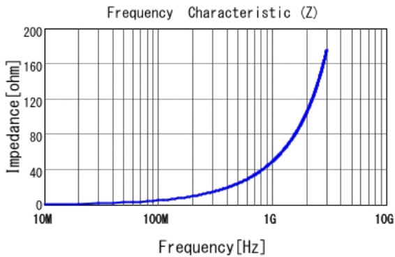
■ LQW15AN7N8C10 |Z|
