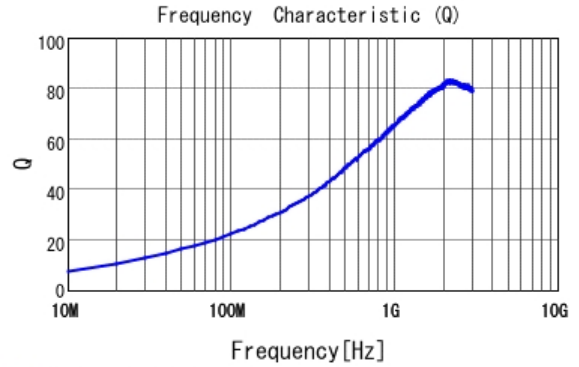
■ LQW15AN7N8C10 Q
