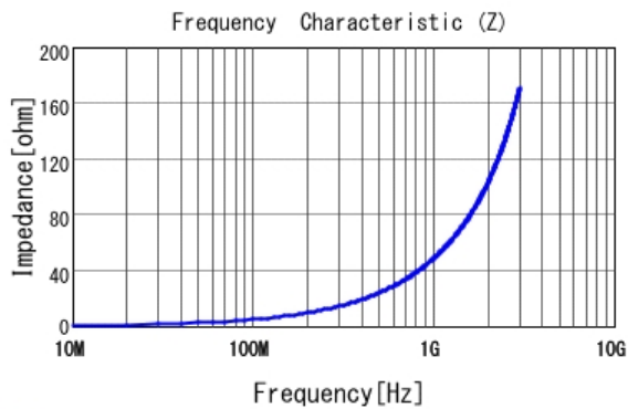
■ LQW15AN7N9C10 |Z|
