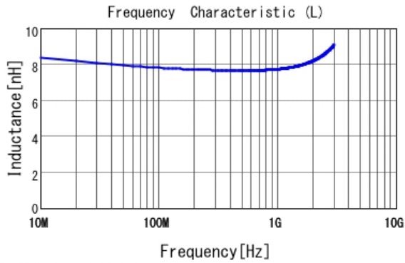
■ LQW15AN7N9C10 L
