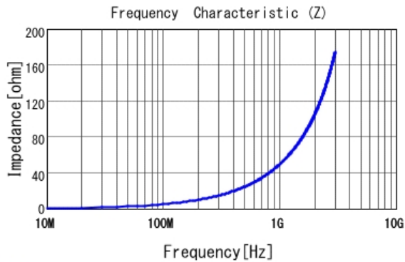
■ LQW15AN8N0C10 |Z|
