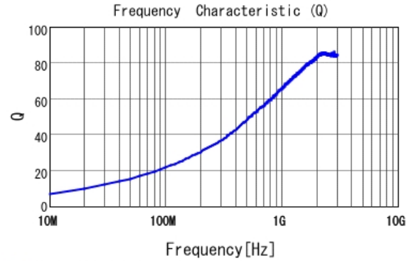
■ LQW15AN8N0C10 Q
