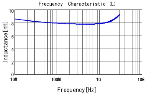
■ LQW15AN8N0C10 L
