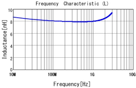
■ LQW15AN8N1C10 L
