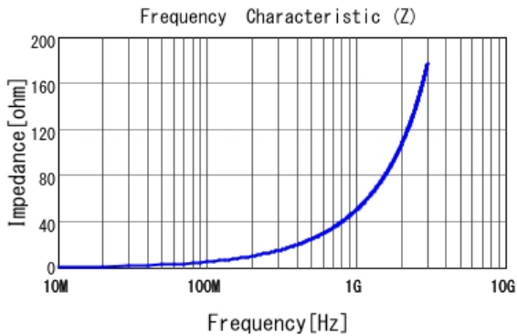
■ LQW15AN8N1C10 |Z|
