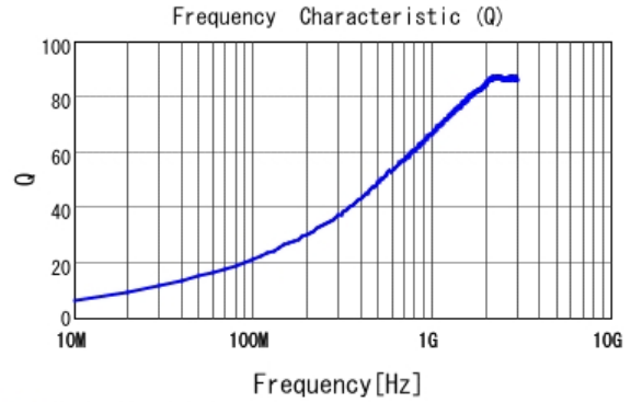
■ LQW15AN8N1C10 Q
