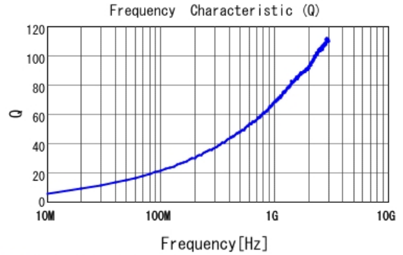
■ LQW15AN8N2G00 Q
