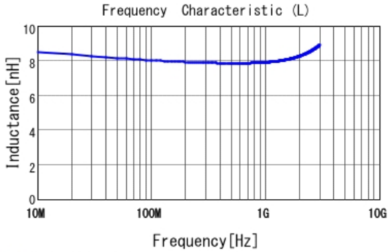
■ LQW15AN8N2G00 L
