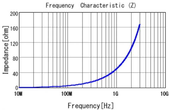
■ LQW15AN8N2G00 |Z|
