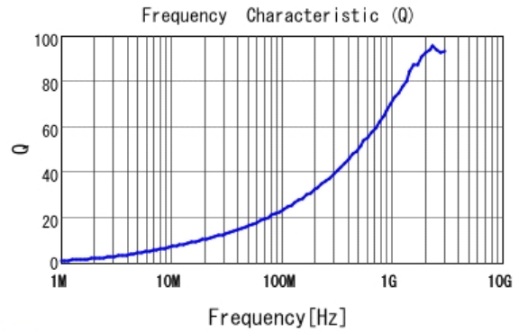
■ LQW15AN8N2G80 Q
