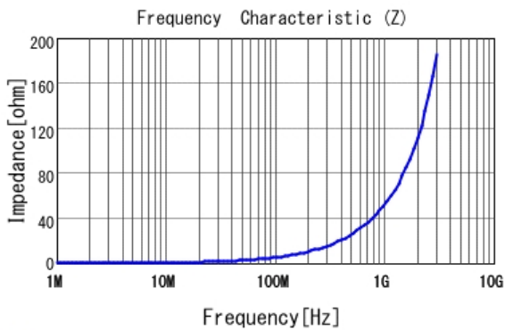
■ LQW15AN8N2G80 |Z|
