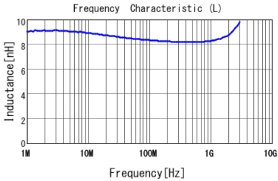
■ LQW15AN8N2G80 L
