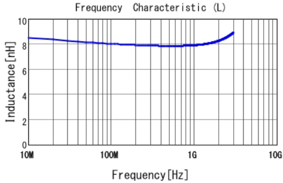
■ LQW15AN8N2J00 L
