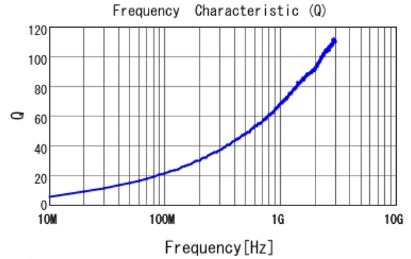
■ LQW15AN8N2J00 Q
