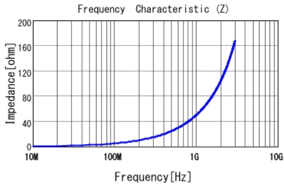
■ LQW15AN8N2J00 |Z|
