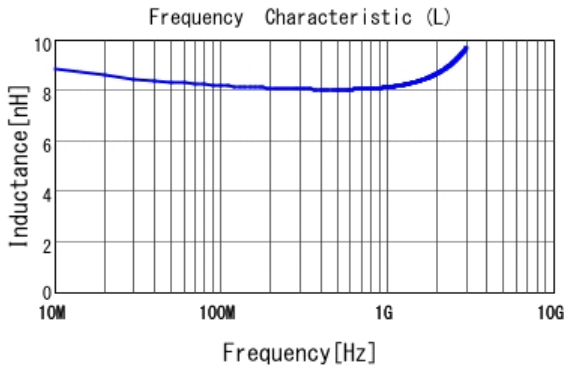
■ LQW15AN8N3C10 L
