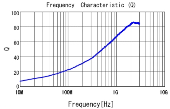
■ LQW15AN8N3C10 Q
