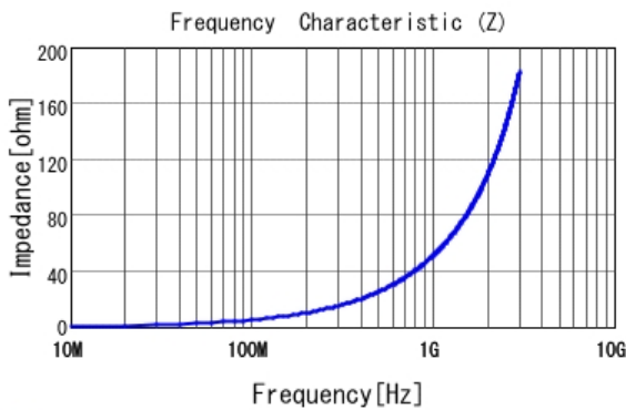
■ LQW15AN8N3C10 |Z|
