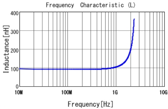
■ LQW15AN91NG00 L
