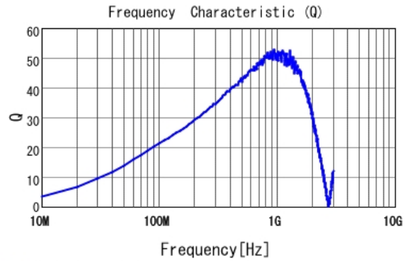
■ LQW15AN91NG00 Q
