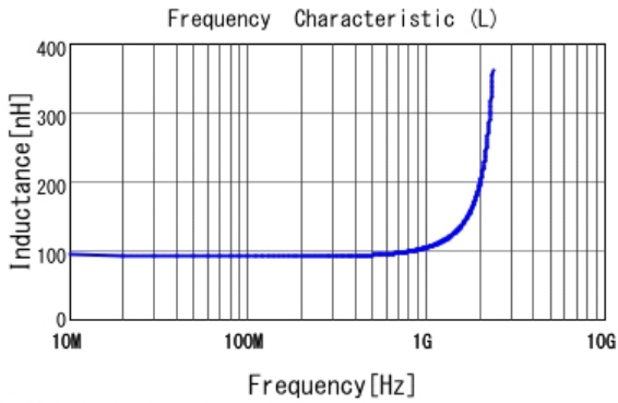
■ LQW15AN91NJ00 L
