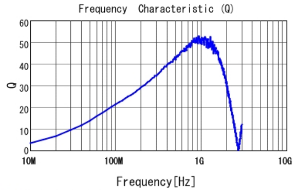
■ LQW15AN91NJ00 Q
